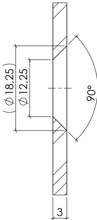
SCHNITT B-B MABSTAB 2 : 1
